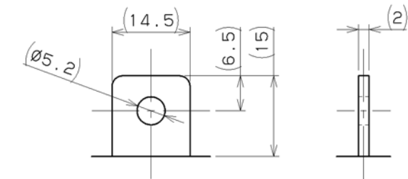
端子部詳細 (1:1)
