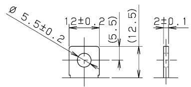
端子部詳細 (1:1)
