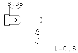
端子部詳細 (1:1)
