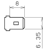
端子部詳細 (1 : 1)
